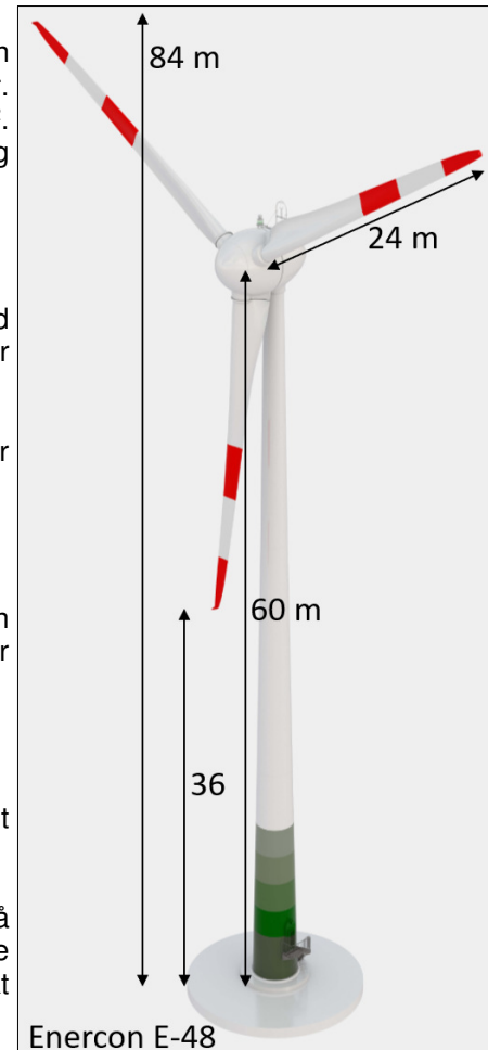
Figur 1. Planlagt vindmølle.
